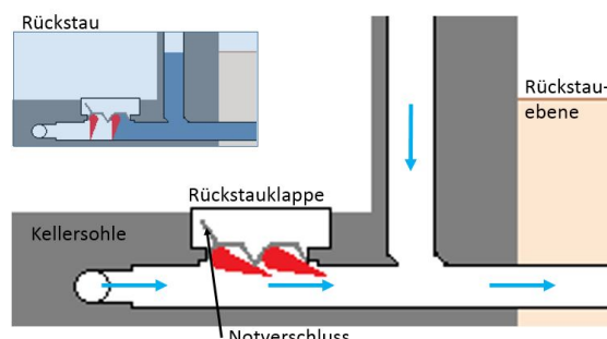
Abb. 20: beispielhafter Rückstauverschluss des Typ 2
