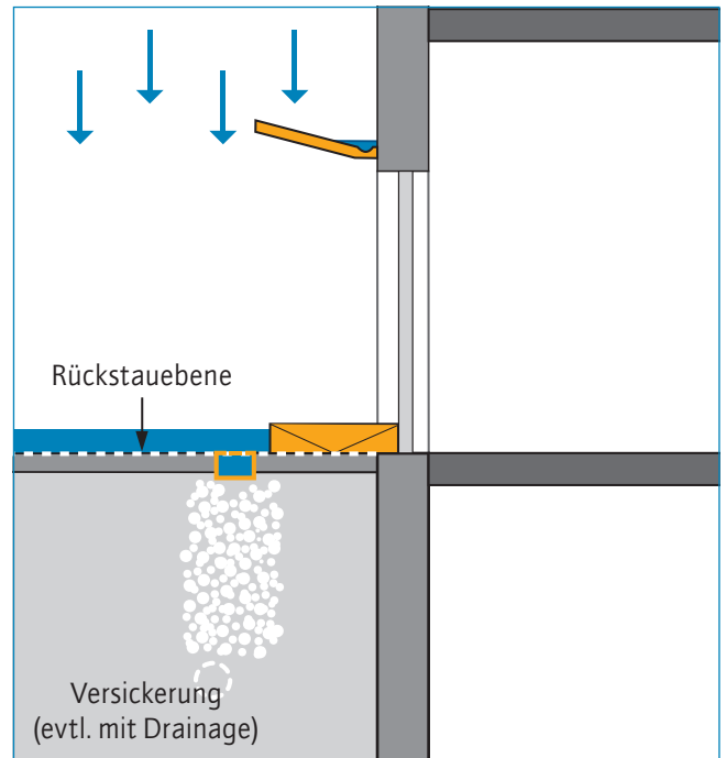
23b Gebäudezugang | RICHTIG
