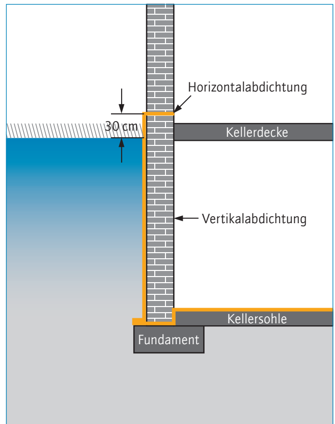
50 Vertikal- und Horizontalabdichtung
