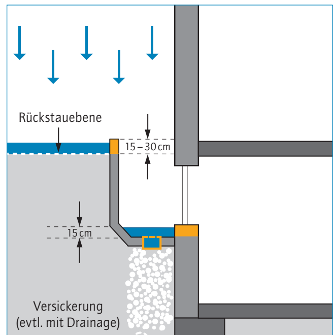
22b Lichtschacht | RICHTIG
