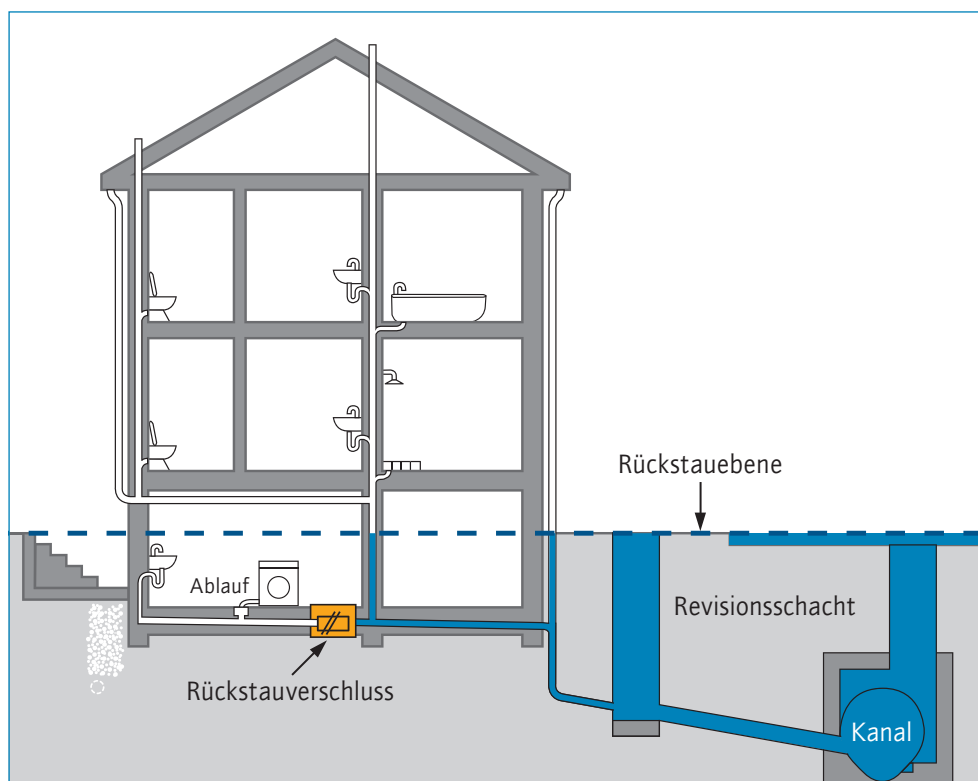
38a Rückstauverschluss | RICHTIG
