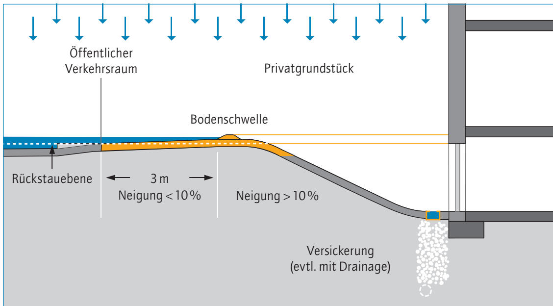
18 Bodenschwelle vor Tiefgaragenzufahrt
