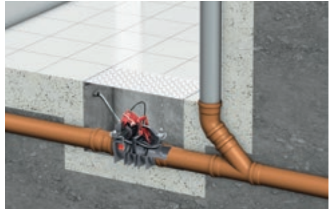
40 Funktionsweise einer Rückstauklappe
