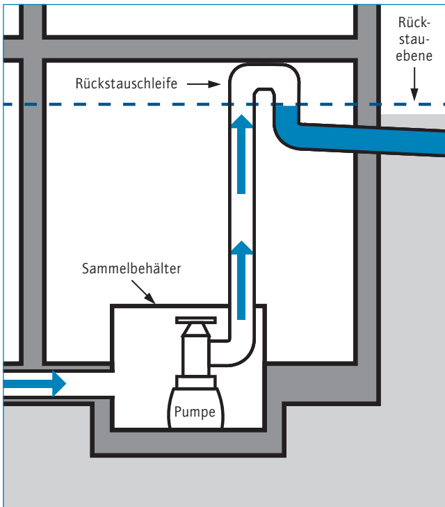
42 Funktionsprinzip einer Hebeanlage
