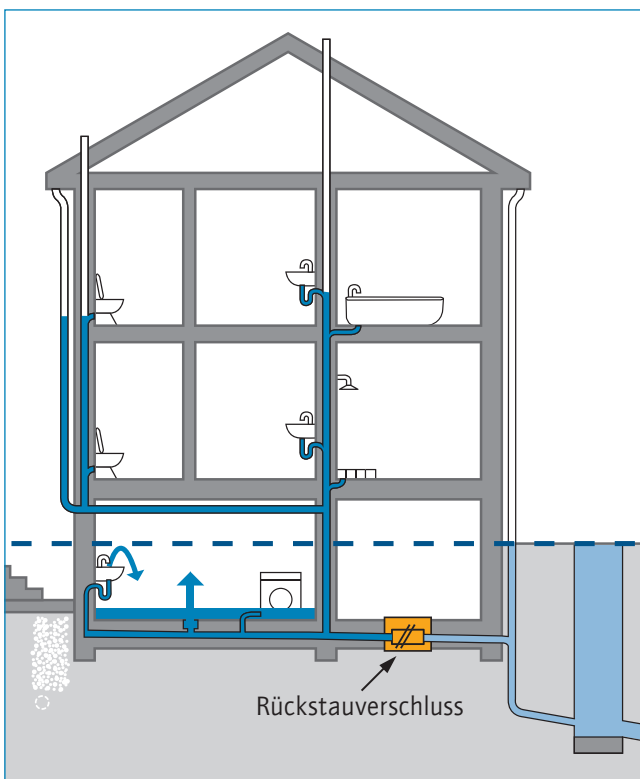
38b Rückstauverschluss | FALSCH
