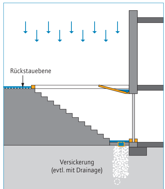
19b Kellertreppe | RICHTIG
