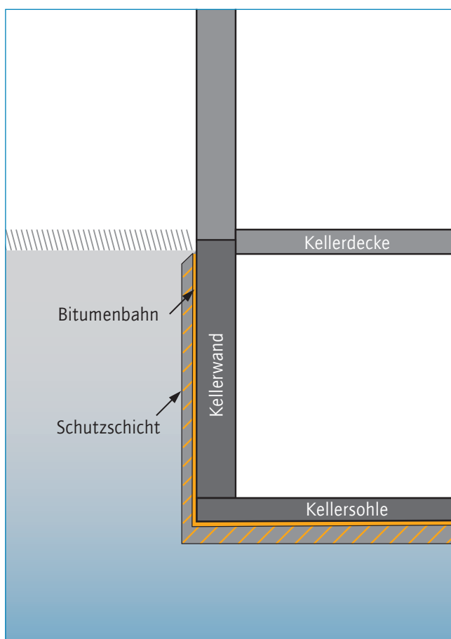
51a Schwarze Wanne
