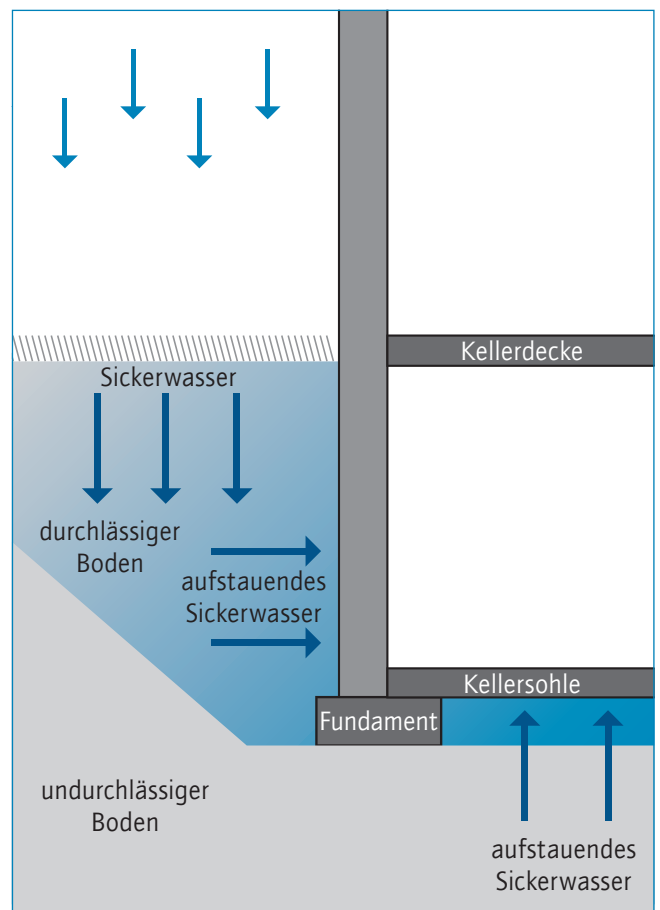
49b Aufstauendes Sickerwasser
