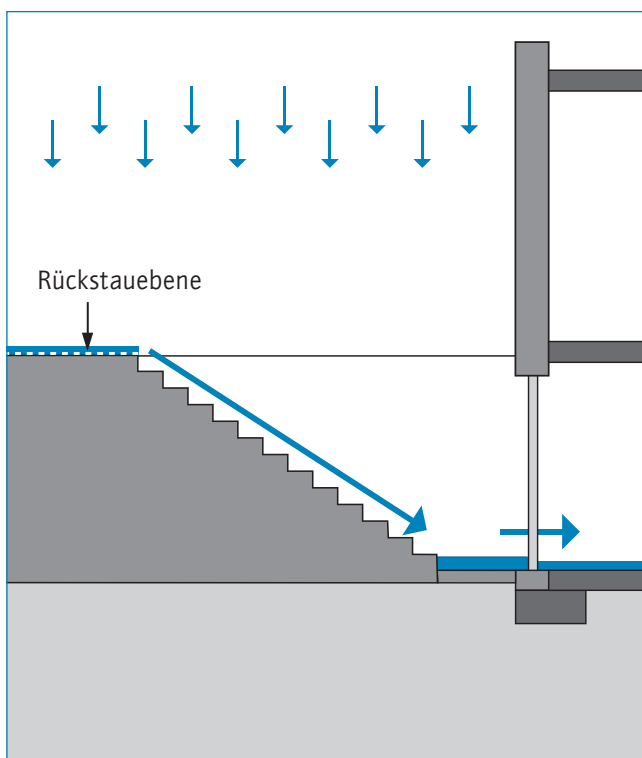
19a Kellertreppe | FALSCH
