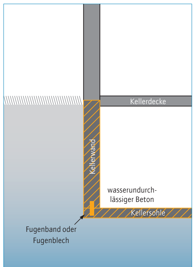
51b Weiße Wanne
