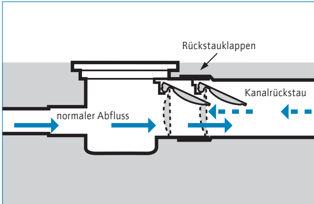
39 Funktionsweise einer Rückstauklappe
