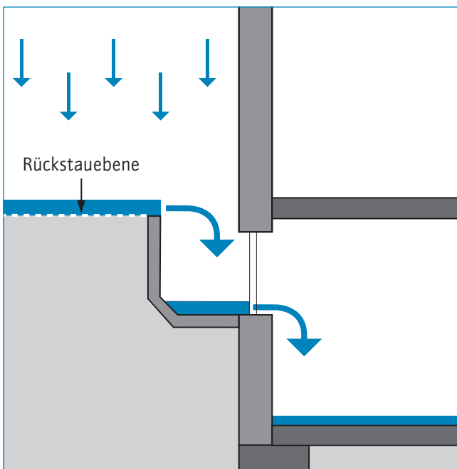
22a Lichtschacht | FALSCH
