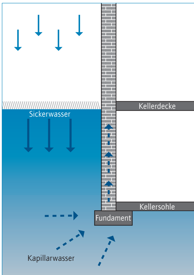
49a Nichtstauendes Sickerwasser
