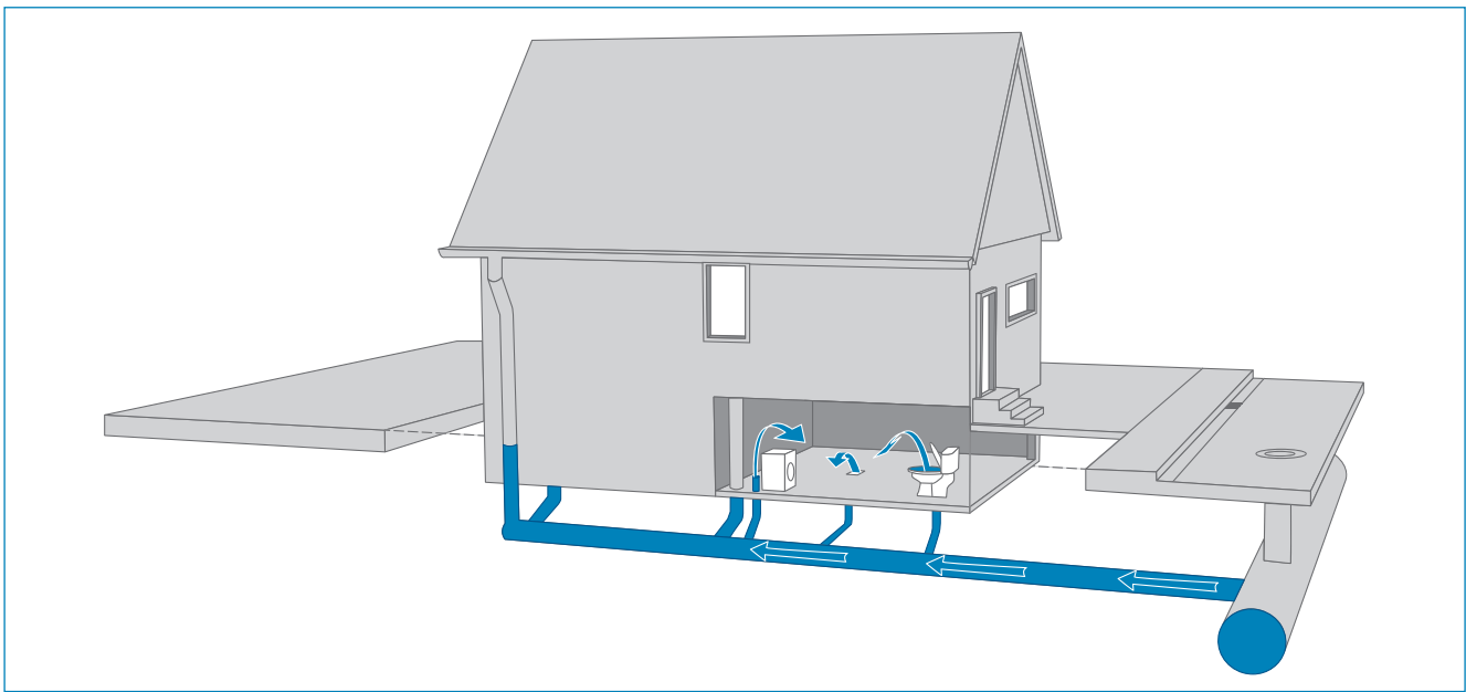
35 Eintrittswege bei Rückstau aus der Kanalisation
