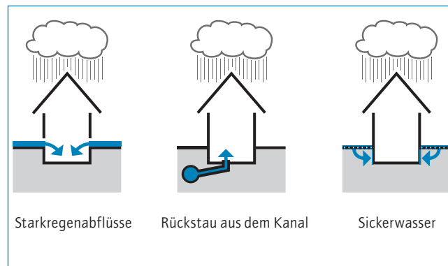
4b Überflutungsgefahren bei Starkregen
