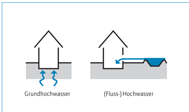
4a Überflutungsgefahren nahe Gewässern*
