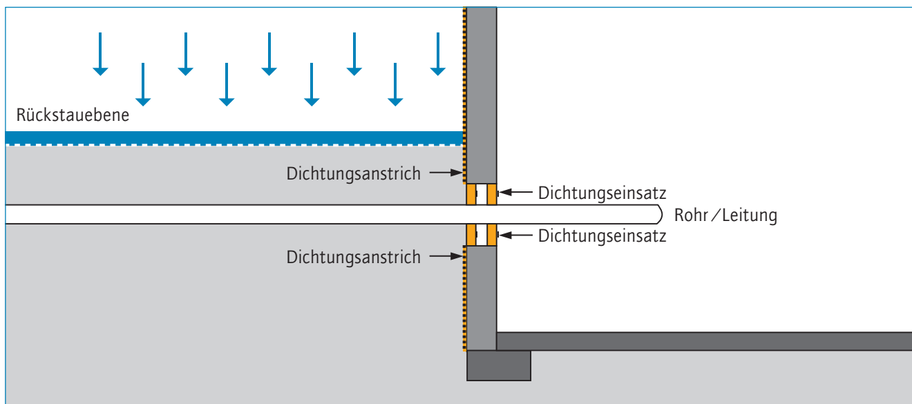
29 Abdichtung von Rohrleitungen
