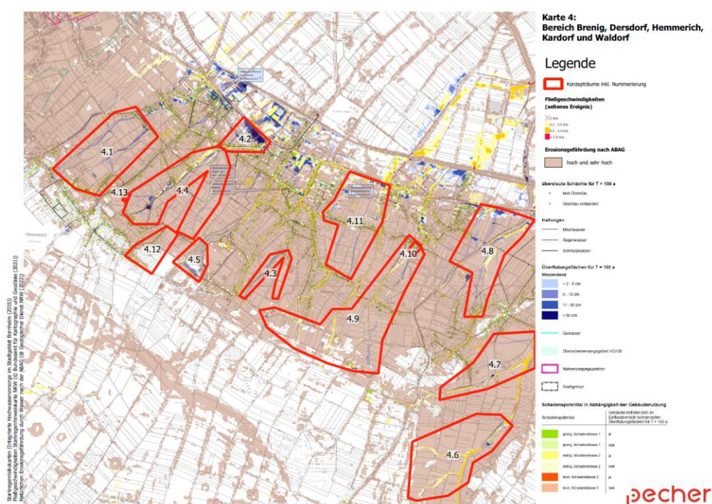
Bild 21 Übersichtskarte der kombinierten Betrachtung der Starkregenrisikokarten der Stadt Bornheim mit Überflutungsflächen (Blautöne), der Starkregenhinweiskarten des Landes NRW für Fließgeschwindigkeiten eines Starkregenereignisses mit einer Wiederkehrzeit von T = 100 a (gelb, orange, rot), sowie der Natürlichen Erosionsgefährdung durch Wasser nach ABAG für eine hohe und sehr hohe Gefährdung (braun)
