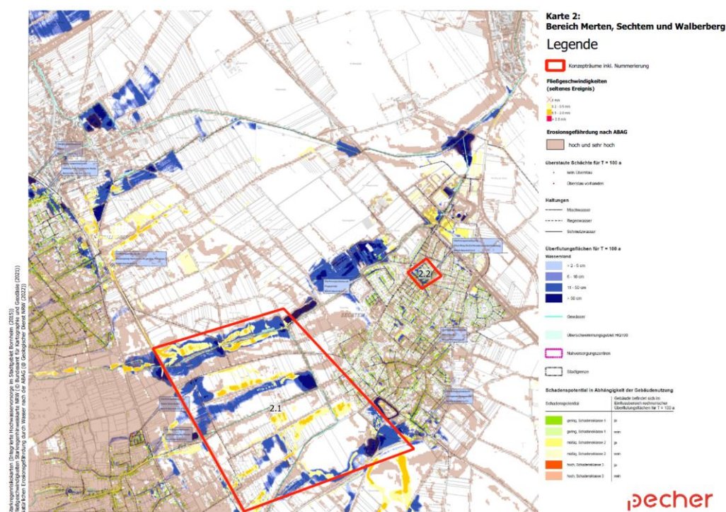
Bild 17 Übersichtskarte der kombinierten Betrachtung der Starkregenrisikokarten der Stadt Bornheim mit Überflutungsflächen (Blautöne), der Starkregenhinweiskarten des Landes NRW für Fließgeschwindigkeiten eines Starkregenereignisses mit einer Wiederkehrzeit von T = 100 a (gelb, orange, rot), sowie der Natürlichen Erosionsgefährdung durch Wasser nach ABAG für eine hohe und sehr hohe Gefährdung (braun)
