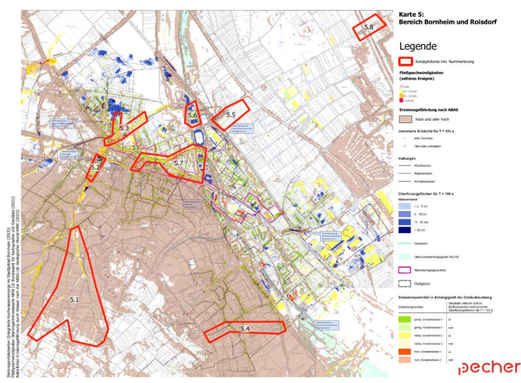
Bild 22 Übersichtskarte der kombinierten Betrachtung der Starkregenrisikokarten der Stadt Bornheim mit Überflutungsflächen (Blautöne), der Starkregenhinweiskarten des Landes NRW für Fließgeschwindigkeiten eines Starkregenereignisses mit einer Wiederkehrzeit von T = 100 a (gelb, orange, rot), sowie der Natürlichen Erosionsgefährdung durch Wasser nach ABAG für eine hohe und sehr hohe Gefährdung (braun)
